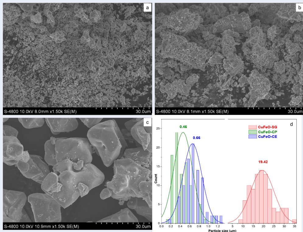
Hình 2: Ảnh FESEM của CuFeO-CE (a), CuFeO-CP (b) và CuFeO-SG (c) samples; (d) phân bố kích thước hạt. [Nguồn: Nhóm tác giả]
