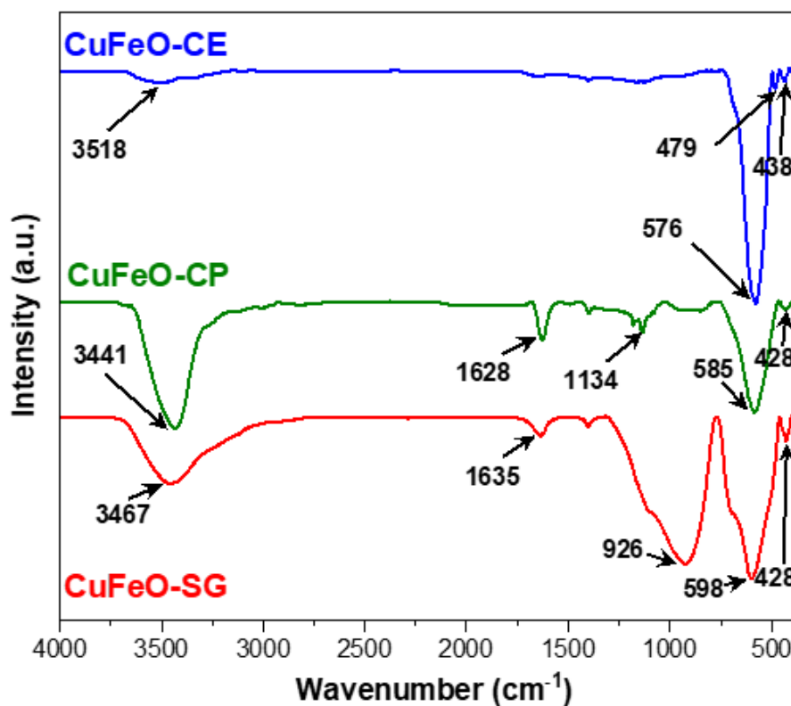
Hình 4: Phổ FTIR của các mẫu CuFeO-CE, CuFeO-CP và CuFeO-SG. [Nguồn: Nhóm tác giả]
